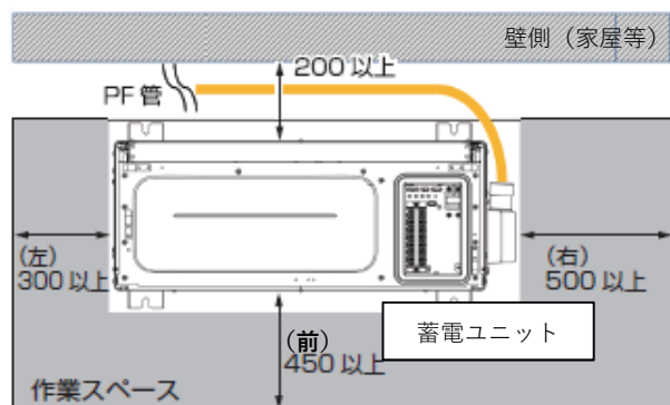
(天板を取り外し、PF管を背面に通した場合の) 上面図
