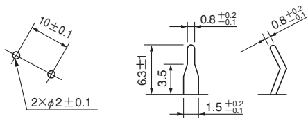
(基板穴寸法)
